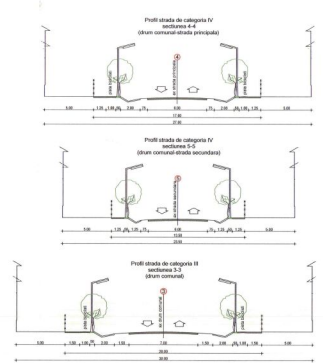
PROFILI CARACTERISTICE DE STRAZI scara 1:2000
